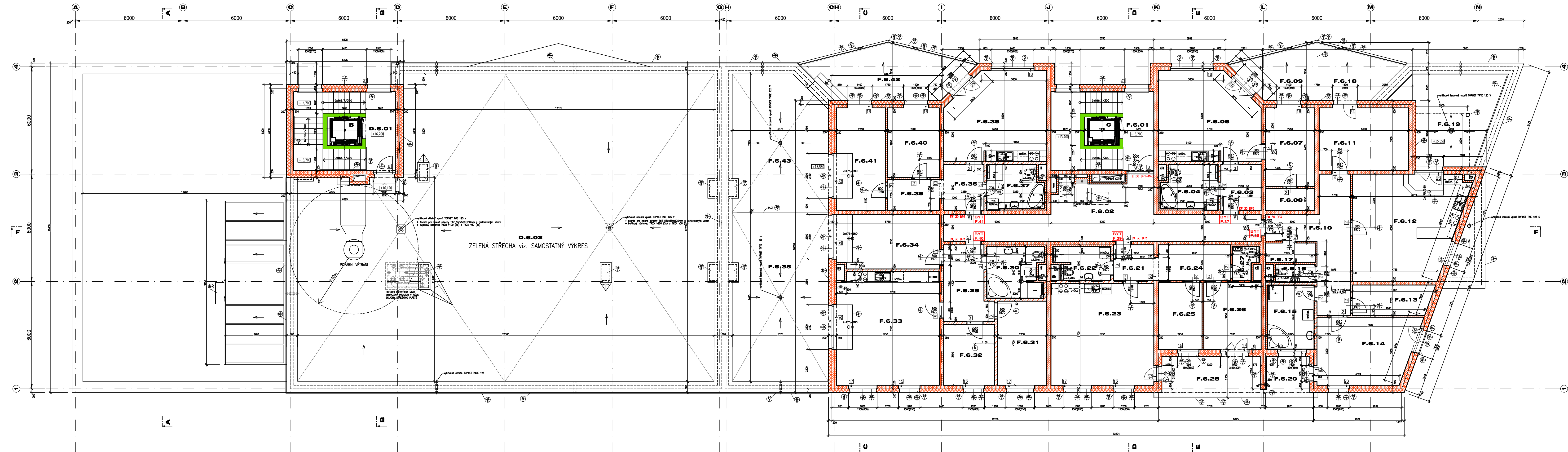
PŮDORYS 6.NP
