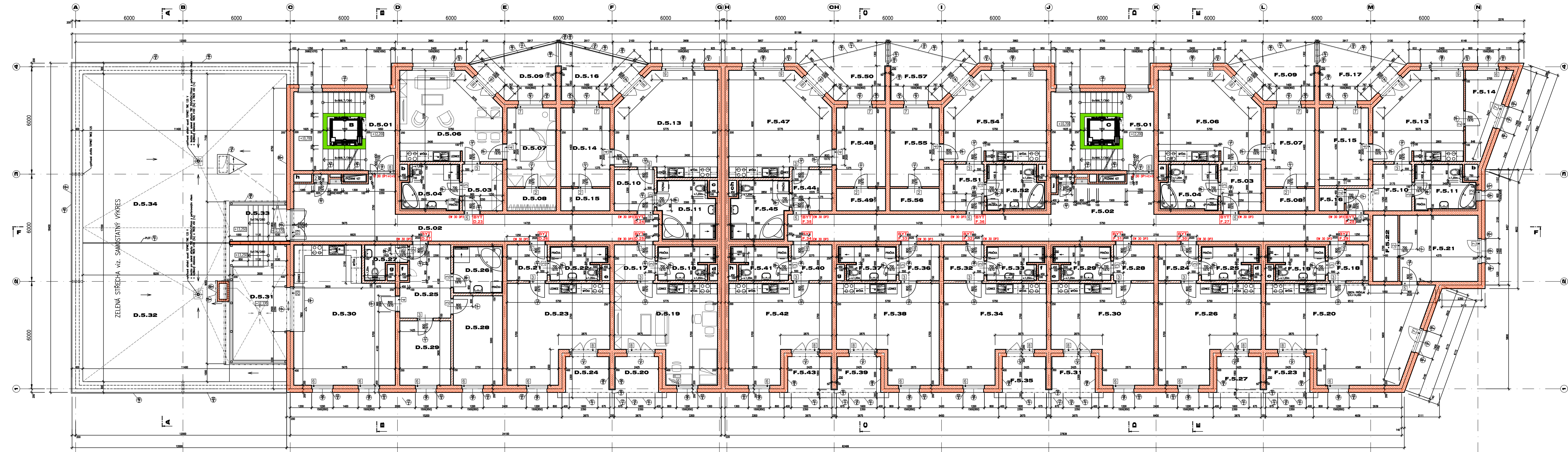
PŮDORYS 5.NP
