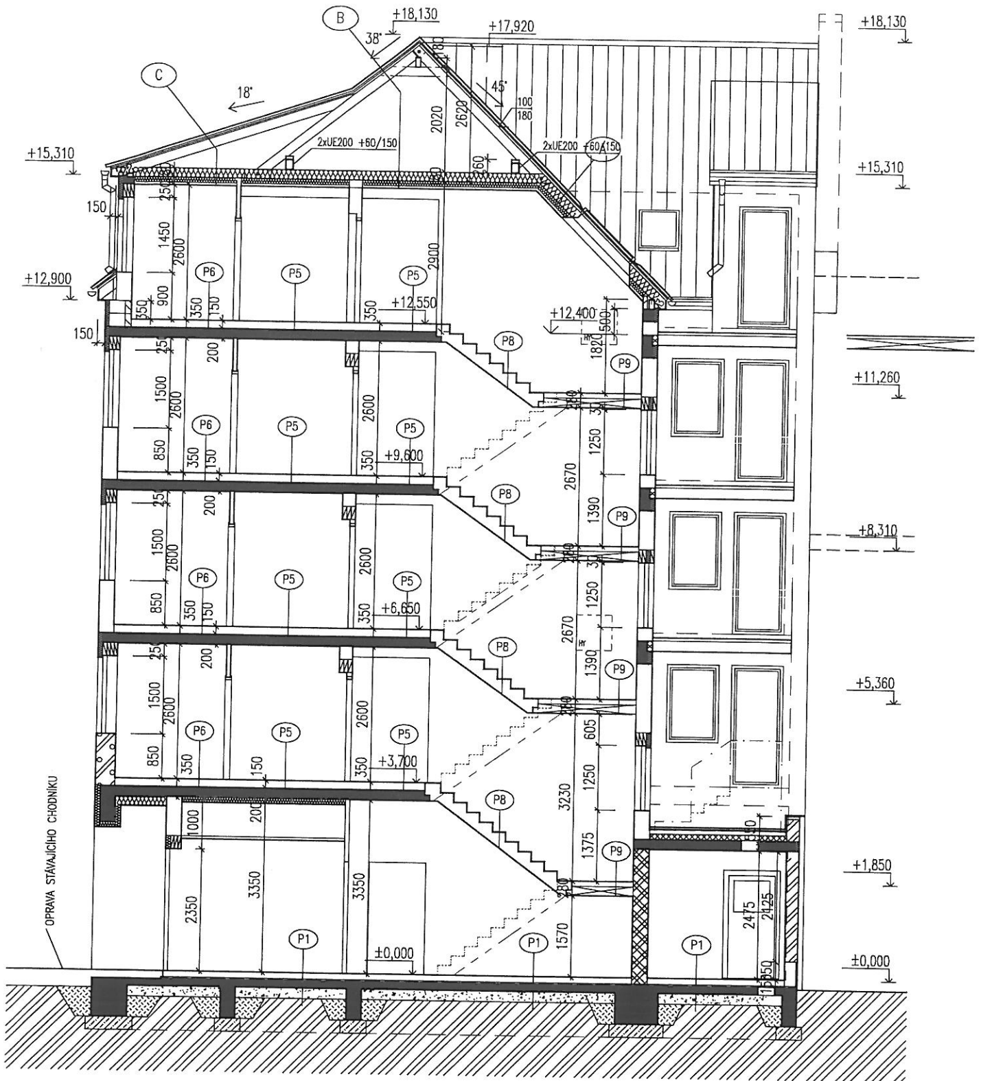
ŘEZ E-E
