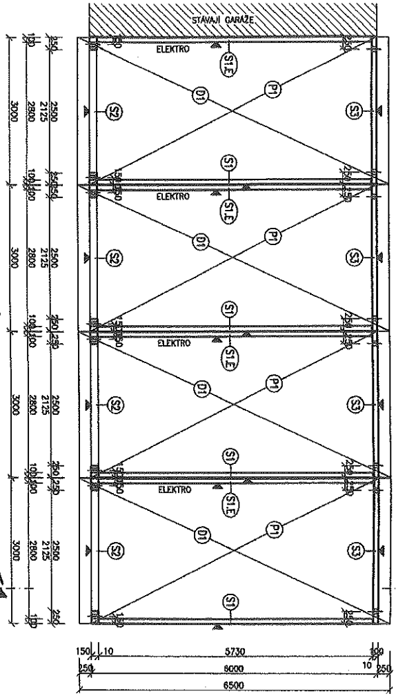
PŮDORŇS 1:50
