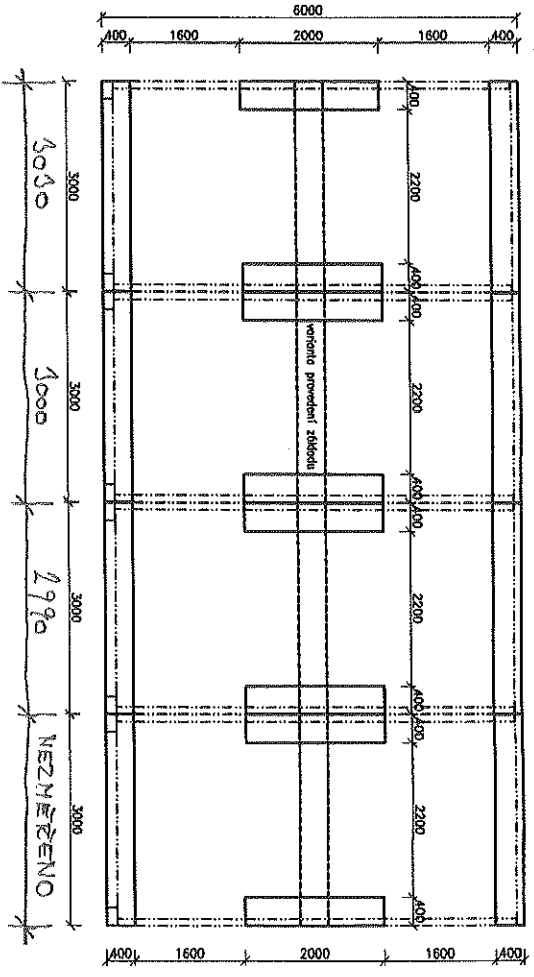
PŮDORŇS-ZAKLADY 1:50
